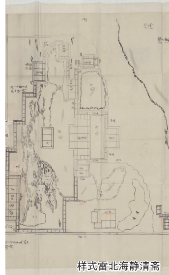
样式雷北海静清斋
